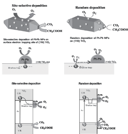
図 18 Pt-Pb 助触媒-TiO 2 界面における励起電子の移動過程：選択担持 (左)、ランダム担持 (右)
